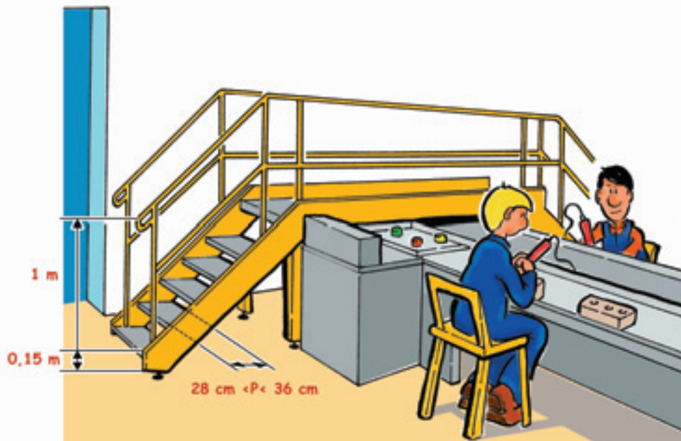
Passerella rialzata protetta al di sopra di una linea di produzione
