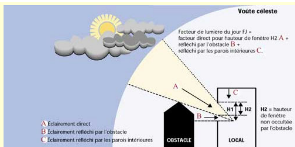
Figure 1 : les composants du facteur de lumière du jour
