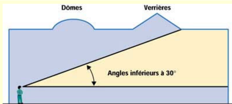
Figure 2 : deux types d'éclairage zénithal
