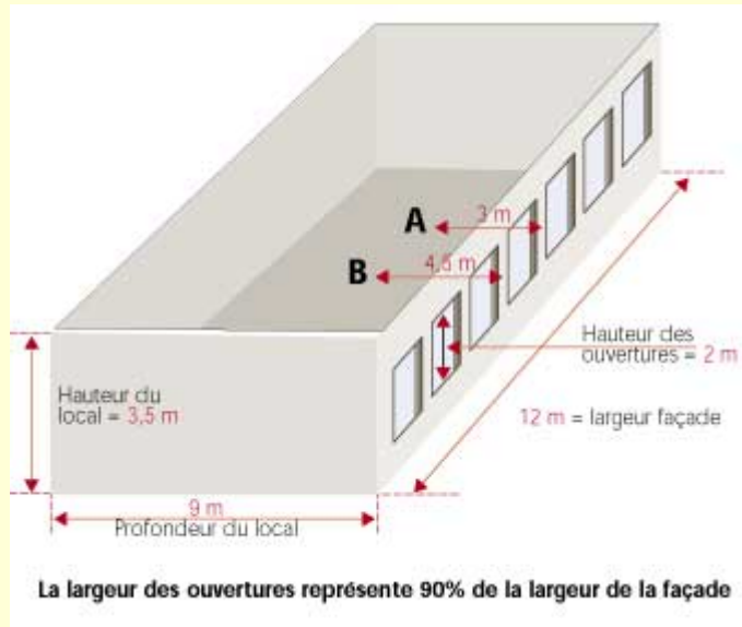
Figure 3 : Évaluation de l'éclairage naturel intérieur d'un local
