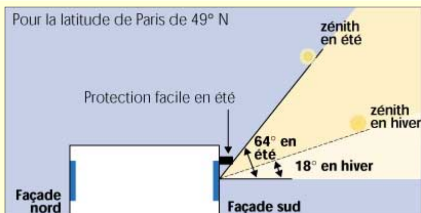
Figure 4 : Orientation conseillée pour les parois vitrées
