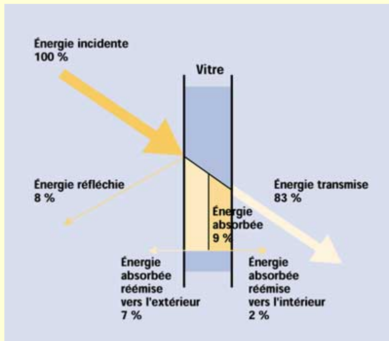
Figure 6 : Facteur solaire des vitrages.
