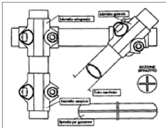
gli elementi costitutivi del ponteggio a giunti e bulloni
