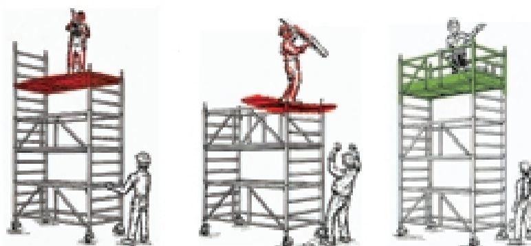
sequenza di montaggio errata (disegni in rosso), solo a montaggio completato (in verde) l'addetto è al riparo dal pericolo di cadere
