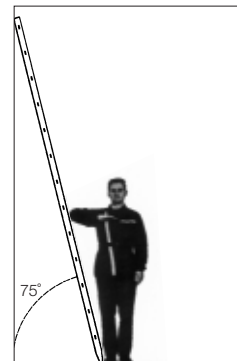
Figura 1: L'angolo d'appoggio corretto (ca. 75°) può essere controllato con la cosiddetta «prova del gomito».
