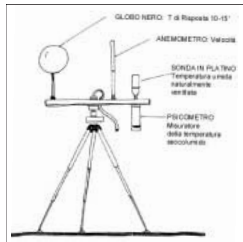
Fig. 27: Centralina microclimatica.
