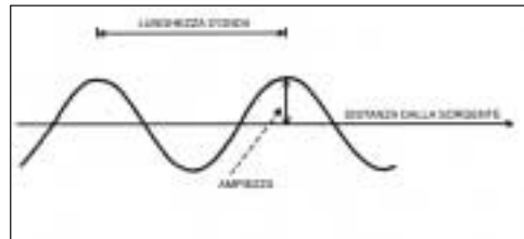
Fig. 9: Rappresentazione di un'onda.
