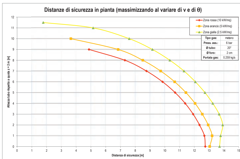
DISTANZA DI SICUREZZA IN PIANTE AL VARIARE DELL'ALTEZZA DELL'ASSE DEL TUBO - TUBO DI DIAMETRO 20" - GAS METANO
