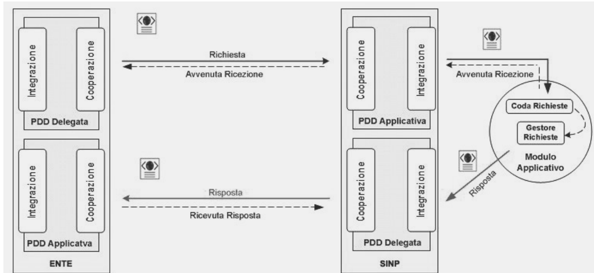
Figura 2 - Profilo Asincrono
